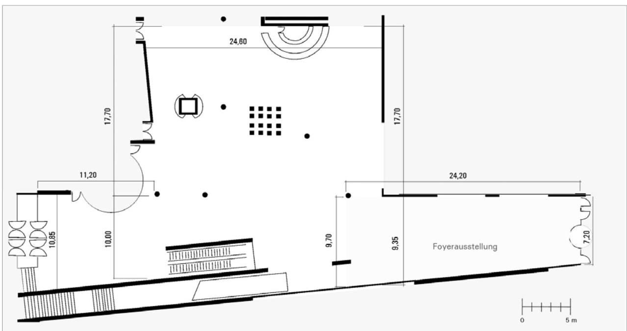
Grundriss M: 1:400
